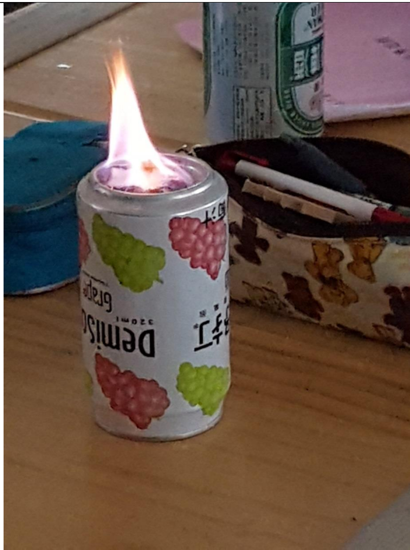
焰色反應。
