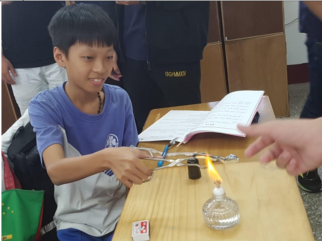
將竹筷用鋁箔紙包起來，以坩鍋鉗夾住在酒精燈下燒烤，最後會得到木炭。
