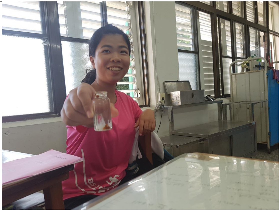
在玻璃瓶中化學花園。
